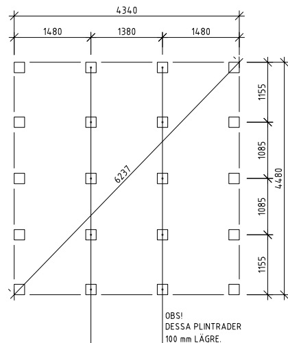
Plintritning
